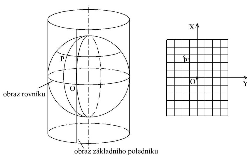
Obr. 7: Ekvidistanční válcové zobrazení v normální poloze
